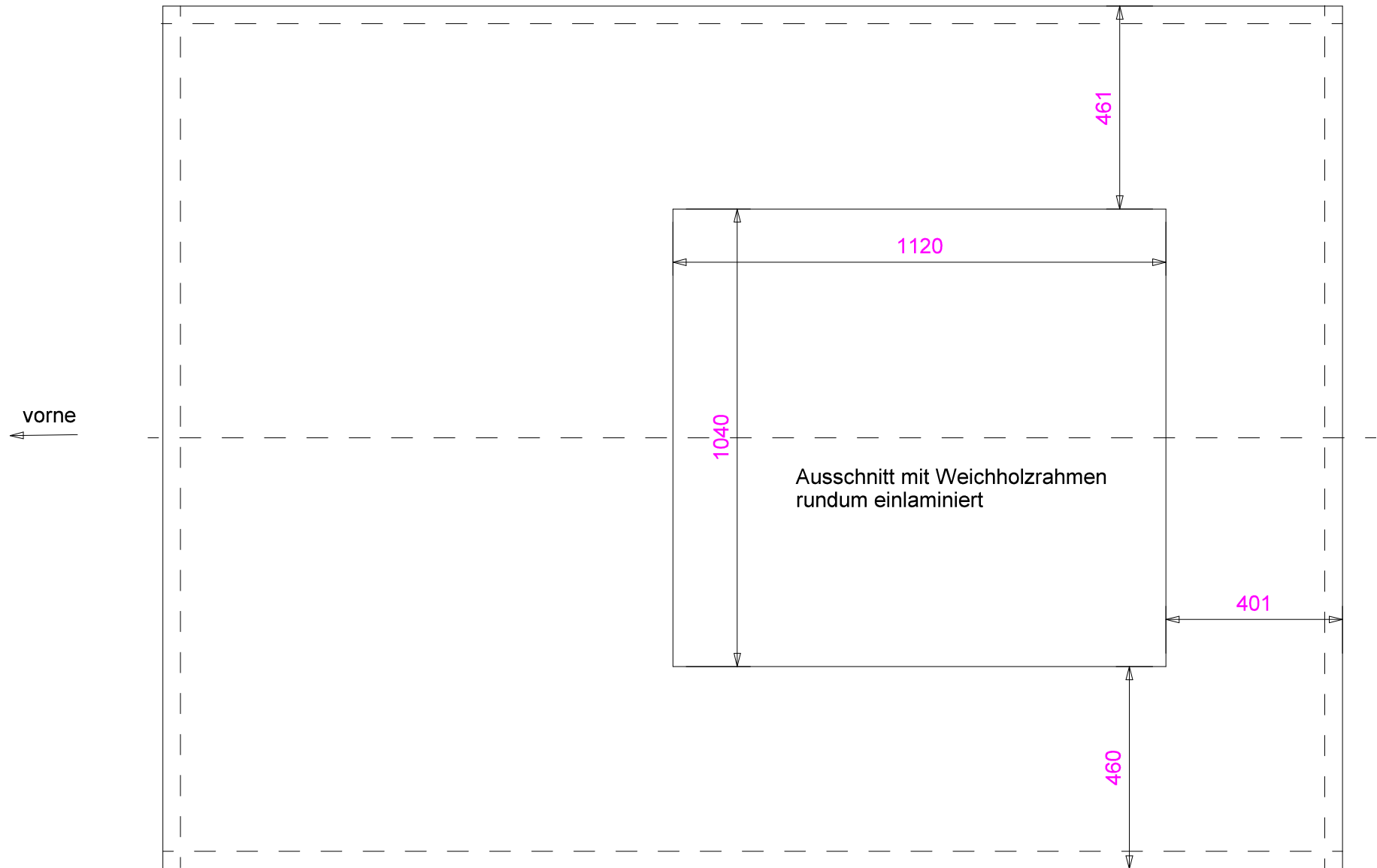
Dachplatte Ansicht von oben, Außenmaß 2700x1960mm
